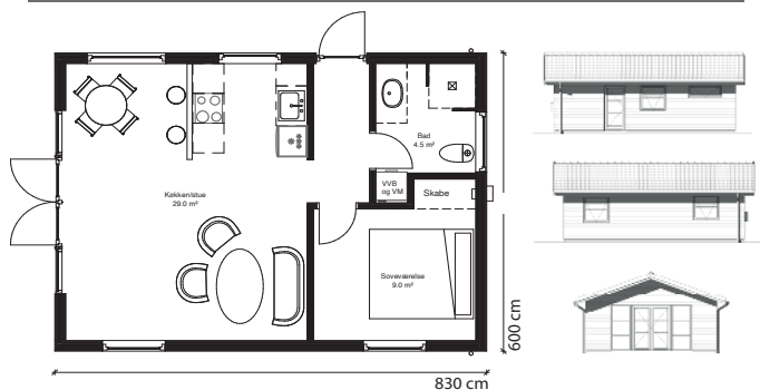
TYPE L50A - 50 m 2
