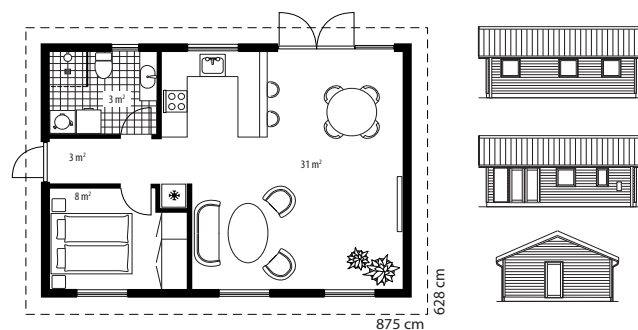
TYPE L55A - 55 m 2
